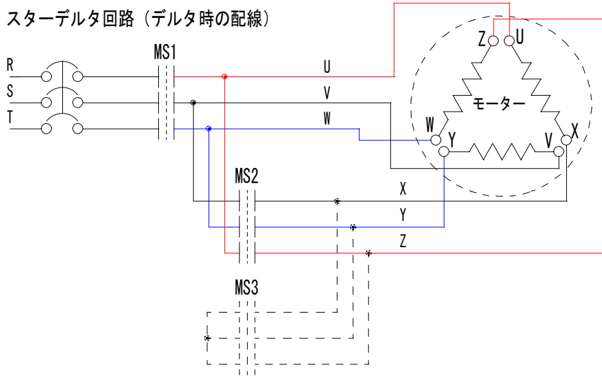
スターデルタ回路から全電圧結線に変更
